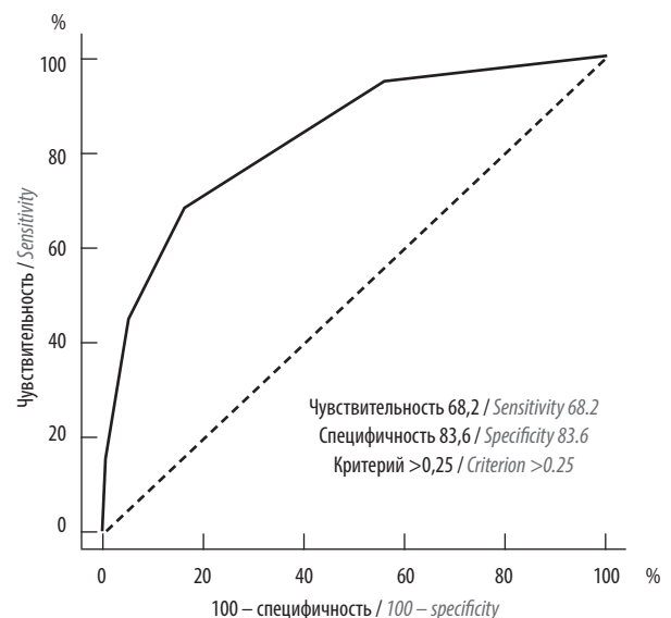
Рис. 3. Характеристики набора маркеров ( MIR9-1 , MIR107 , MIR130b , MIR1258 ) для прогнозирования метастазирования почечно-клеточного рака (площадь под ROC-кривой 0,83)
